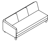
VENS208 208 x 94 H80 81.89"x 37.01" H31.50" IZQ.
